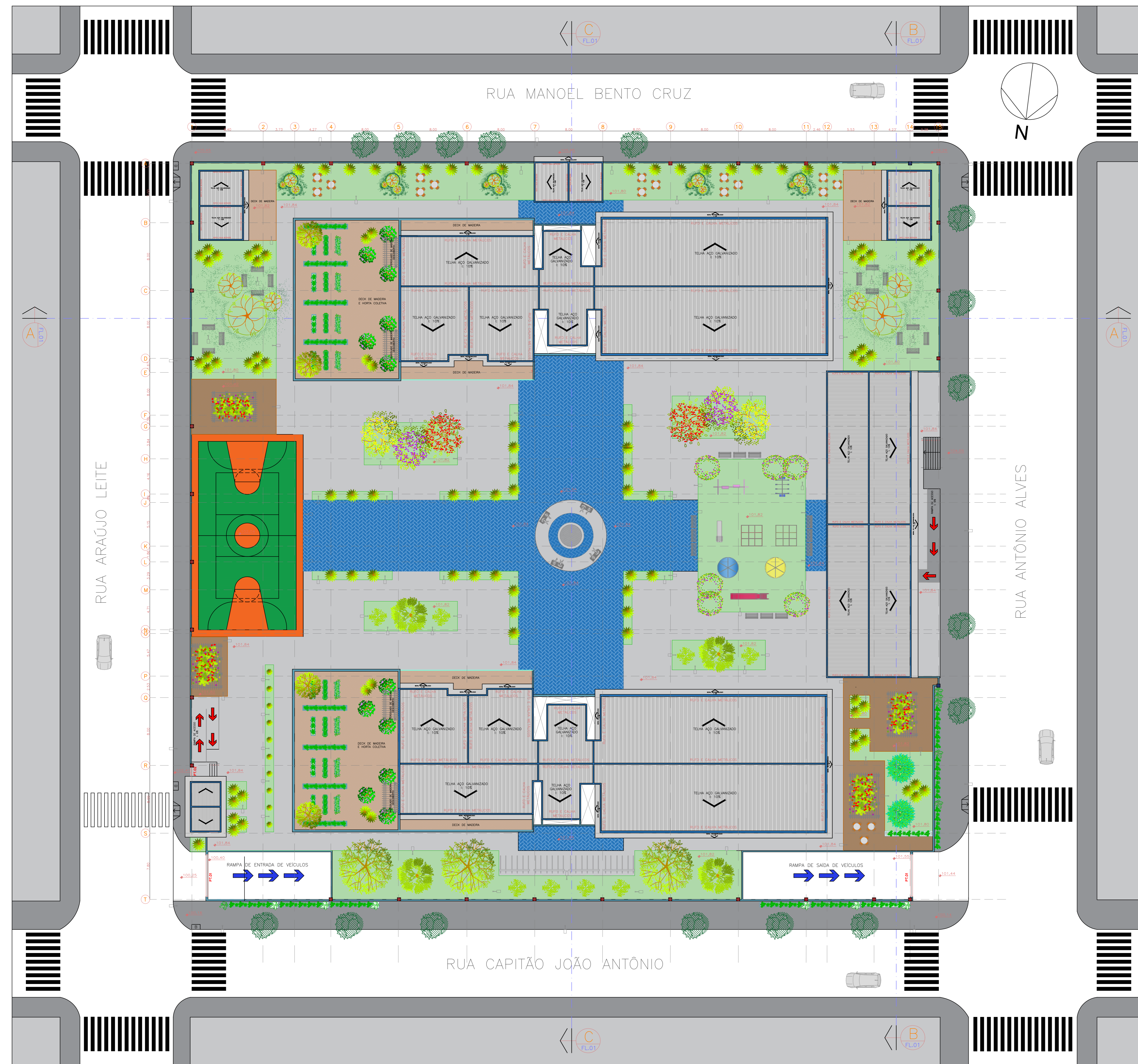
IMPLANTAÇÃO GERAL Esc. 1:200
