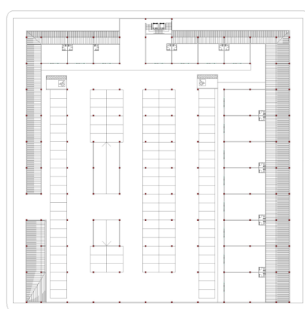
Figura 10. Segundo Subsolo (produção da autora por meio de Eng, Lincoln A. Queiroz)
