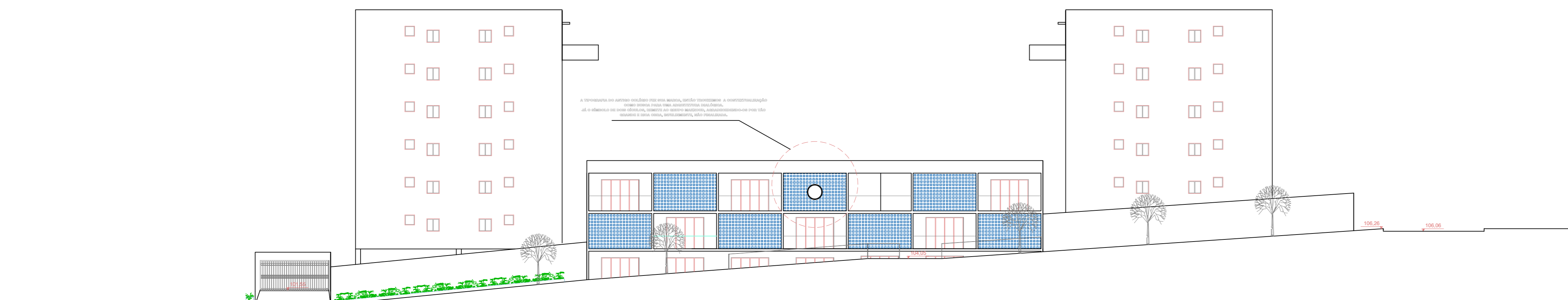
ELEVAÇÃO PELA RUA ANTÔNIO ALVES Esc. 1:200
