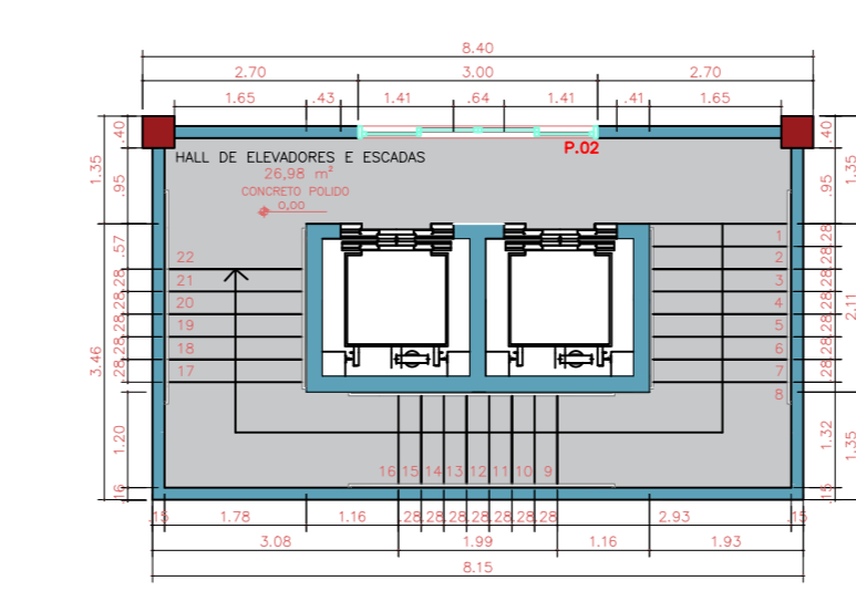
ENTRADA PARA SUBSÓLOS Esc. 1:100
