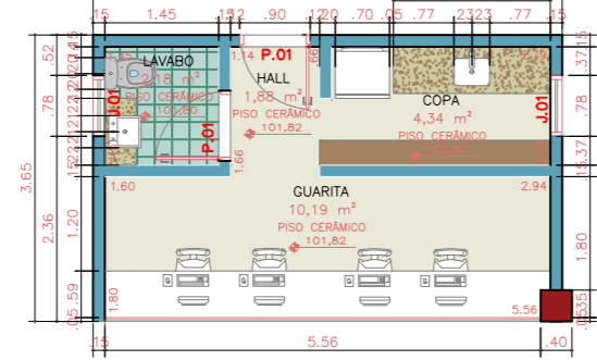
PORTARIA Esc. 1:100
