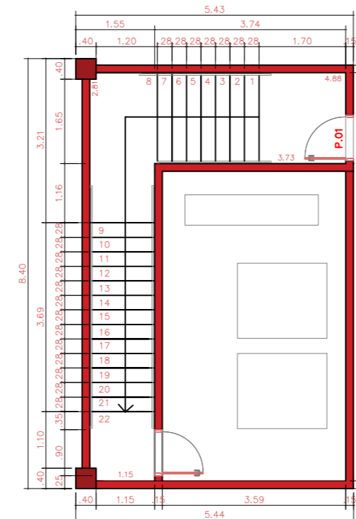
SALA DE AQUECEDORES - 7º SUBSOLO Esc. 1:100 NW 82,82
