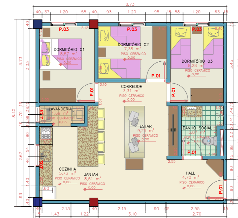
PLANTA TIPOLOGIA 03 Esc. 1:100
