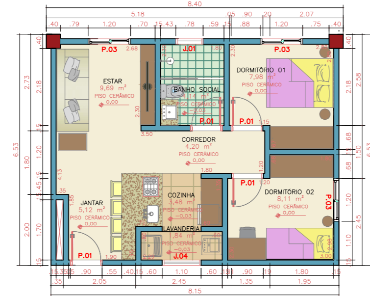
PLANTA TIPOLOGIA 01 Esc. 1:100
