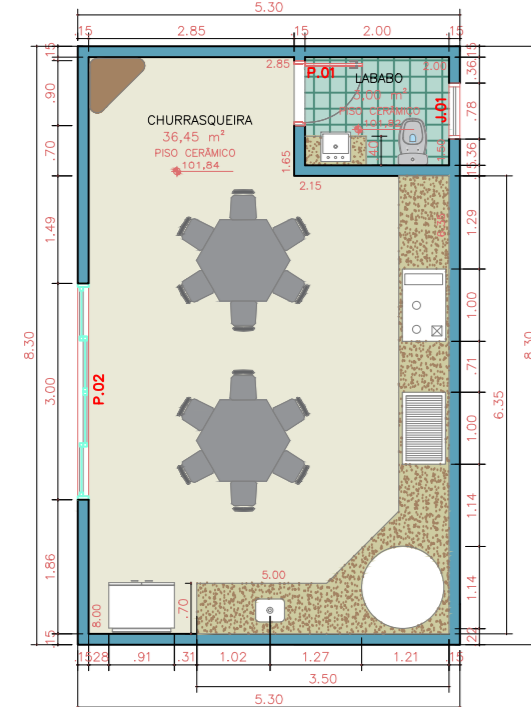
CHURRASQUEIRA 01 Esc. 1:100
