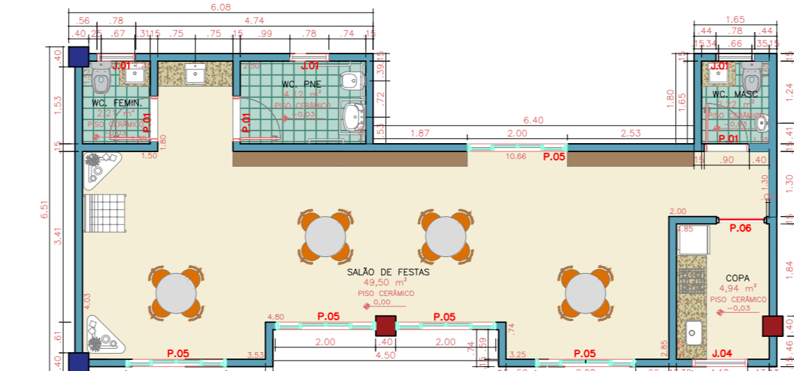
SALÃO DE FESTAS - TORRES HABITACIONAIS (COBERTURA) Esc. 1:100
