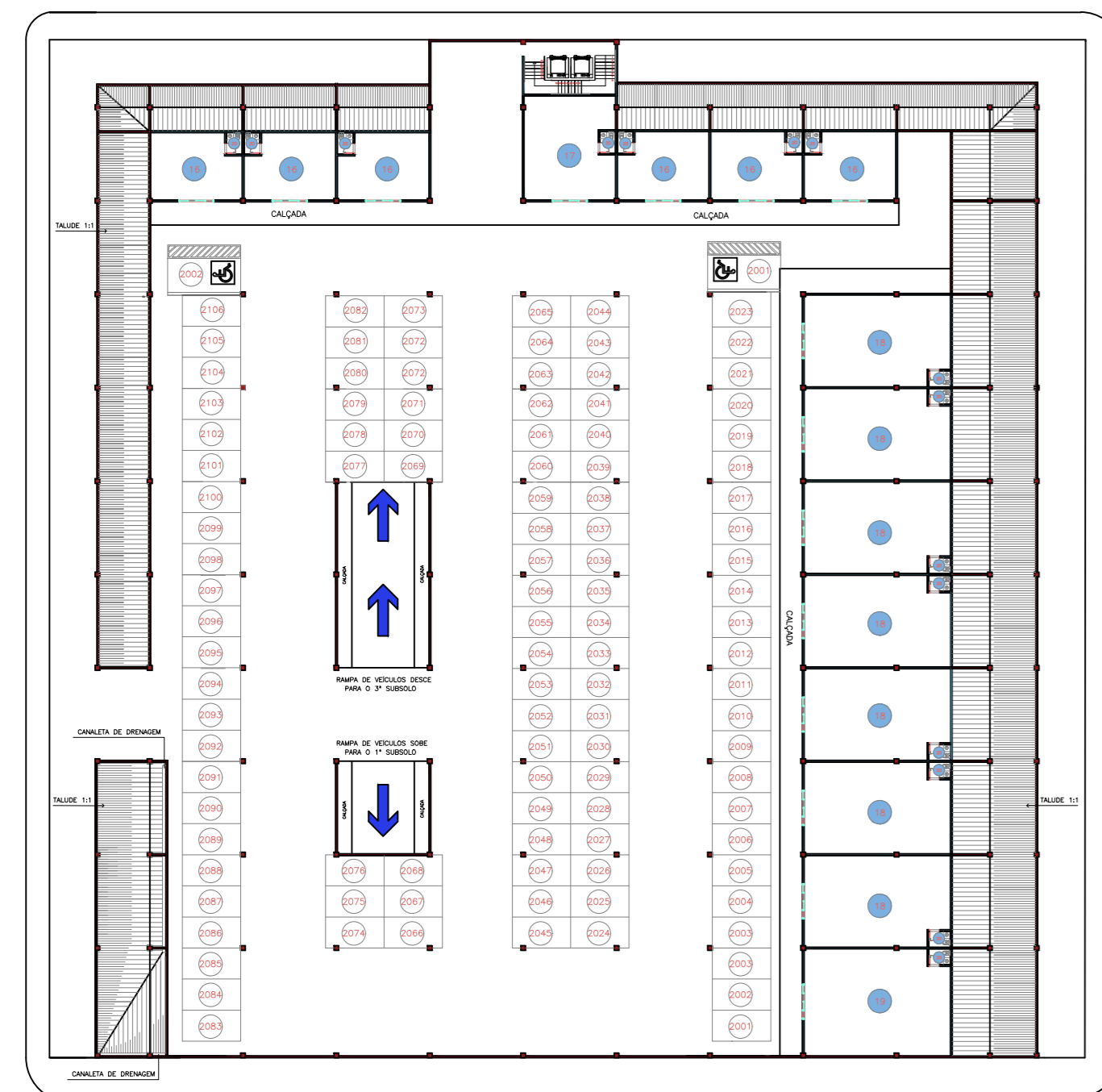
SEGUNDO SUBSOLO Esc. 1:500 NW 94,14
