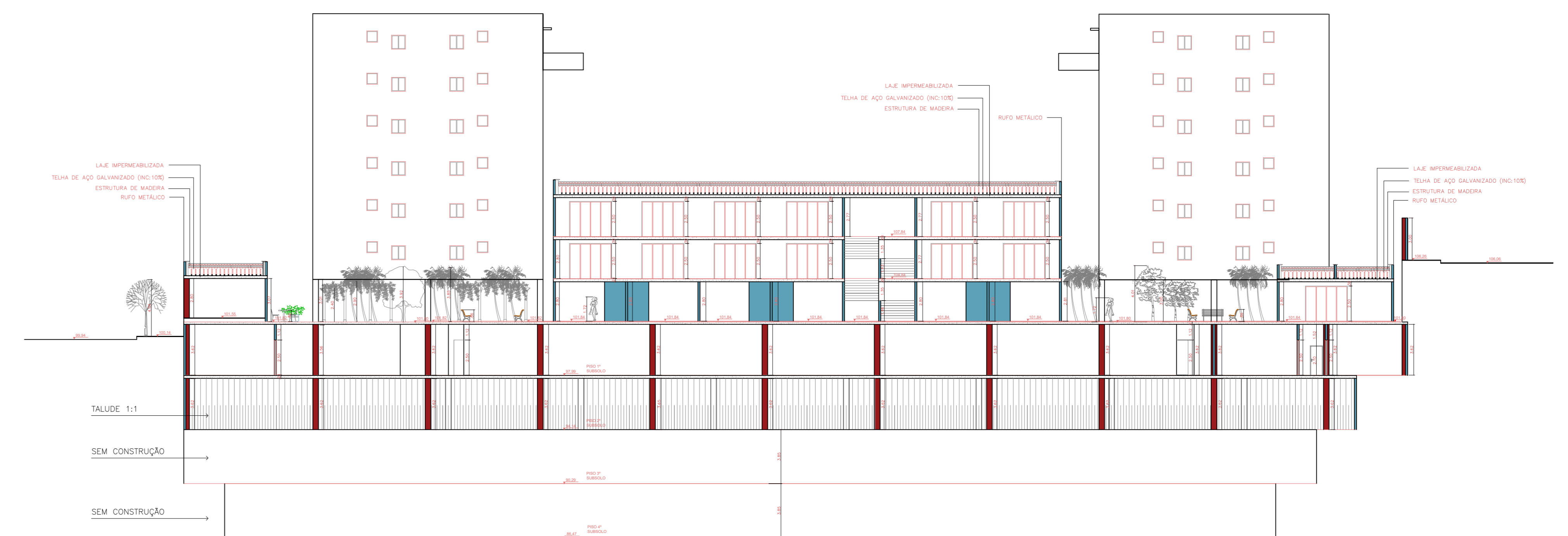
CORTE BB Esc. 1:200
