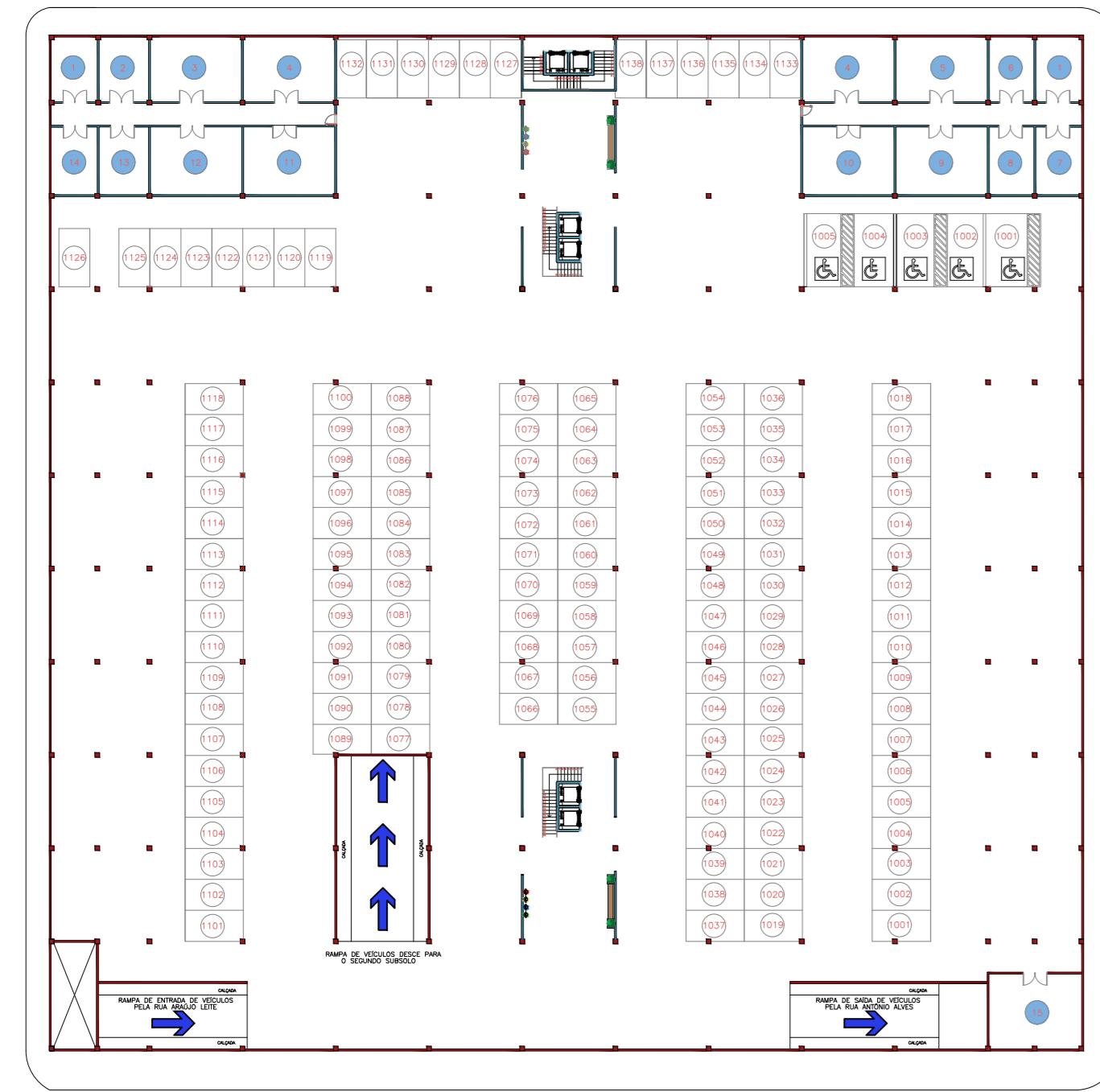
PRIMEIRO SUBSOLO Esc. 1:500 NW 92,39
