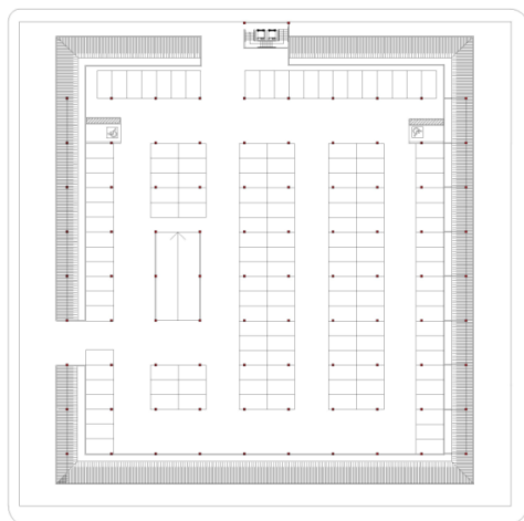
Figura 11. Terceiro Subsolo (produção da autora por meio de Eng, Lincoln A. Queiroz)
