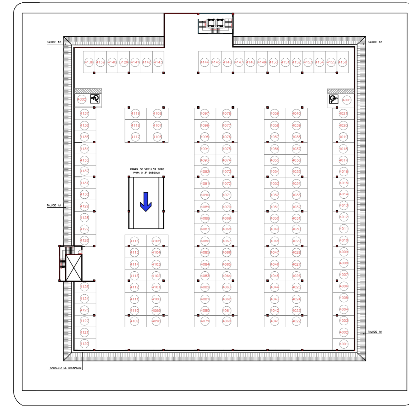
QUINTO SUBSOLO Esc. 1:500 NW 86,47
