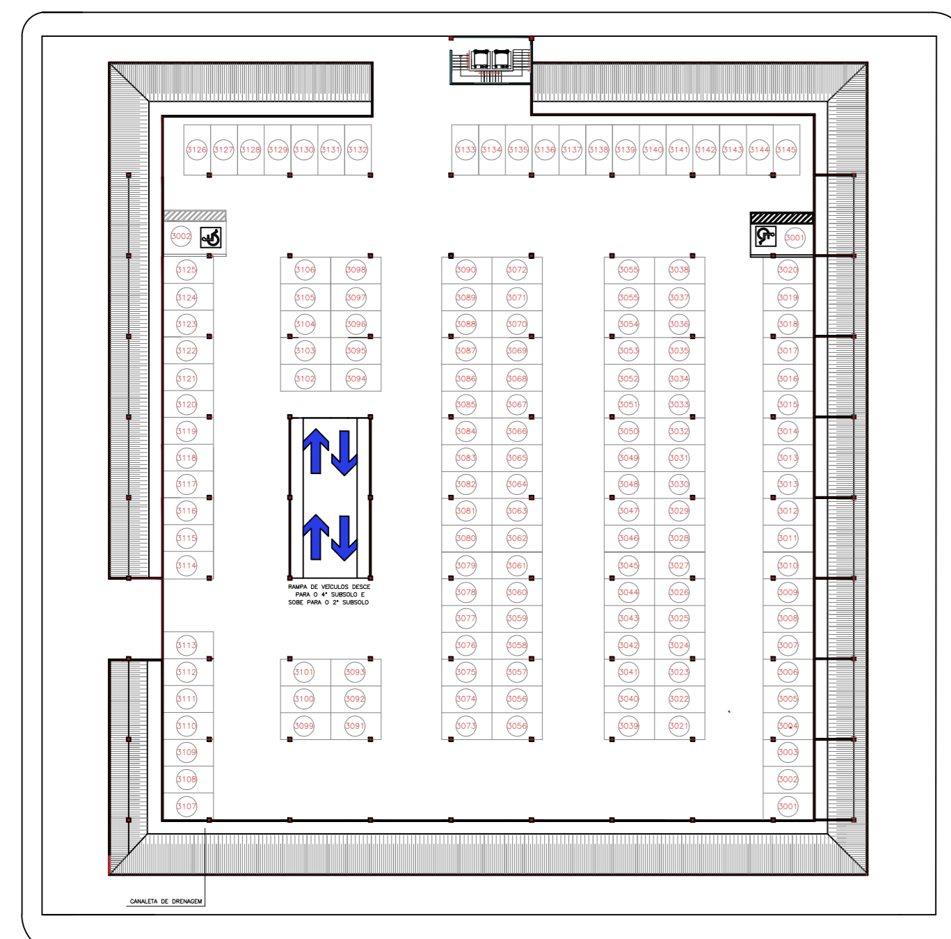
TERCEIRO SUBSOLO Esc. 1:500 NW 90,29
