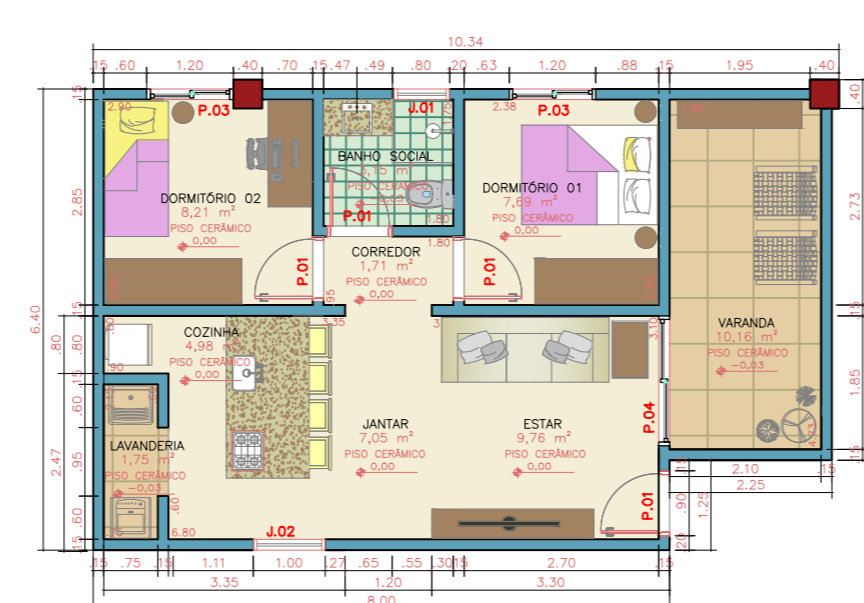
PLANTA TIPOLOGIA 02 Esc. 1:100
