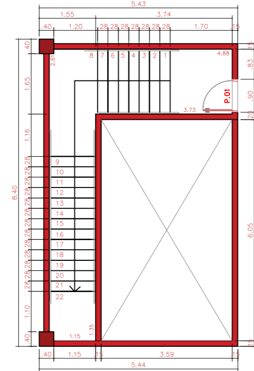
ENTRADA PARA A SALA DE AQUECEDORES - 4º SUBSOLO Esc. 1:100
