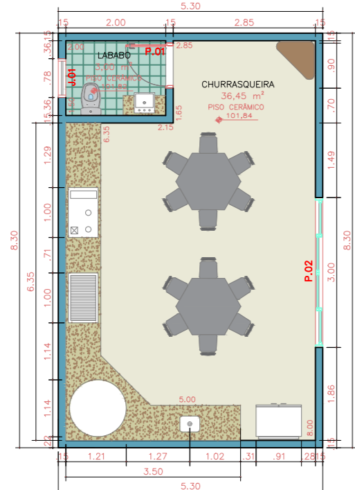
CHURRASQUEIRA 02 Esc. 1:100
