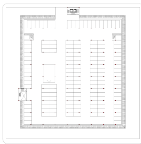
Figura 12. Quarto Subsolo (produção da autora por meio de Eng, Lincoln A. Queiroz)
